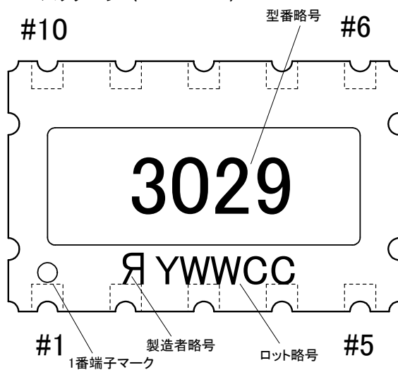
C2パッケージ:(TOP VIEW)
