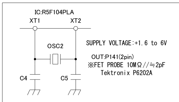
図1 調査回路図
